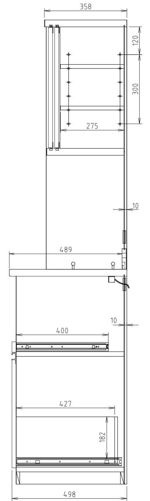
プレファ W140HMオープン
