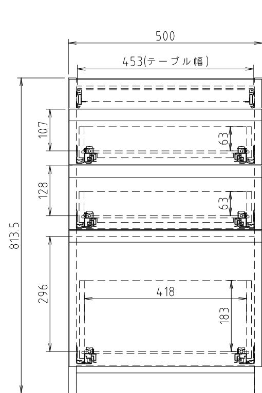
D450タイプ (Sタイプ)
