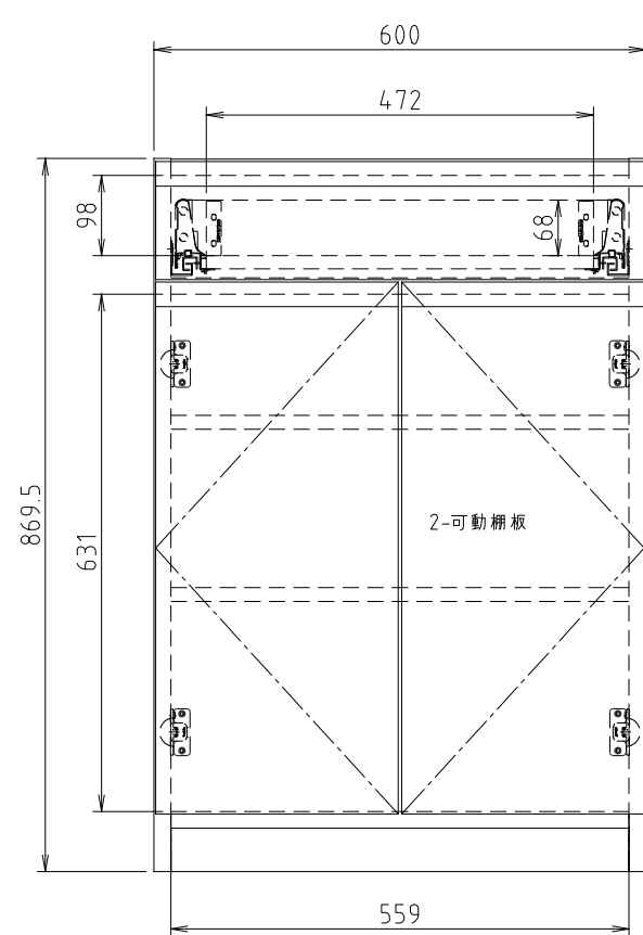
D450タイプ (Sタイプ)
